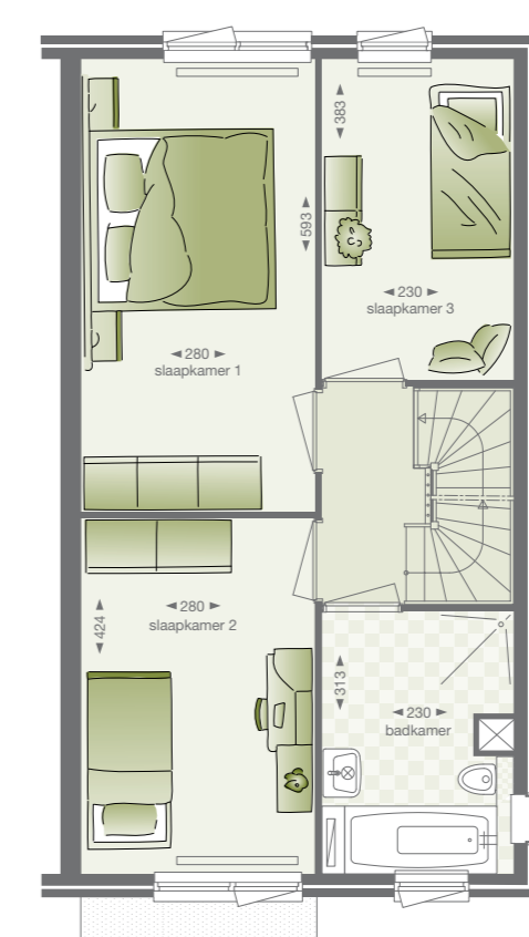
Eerste verdieping - K1
