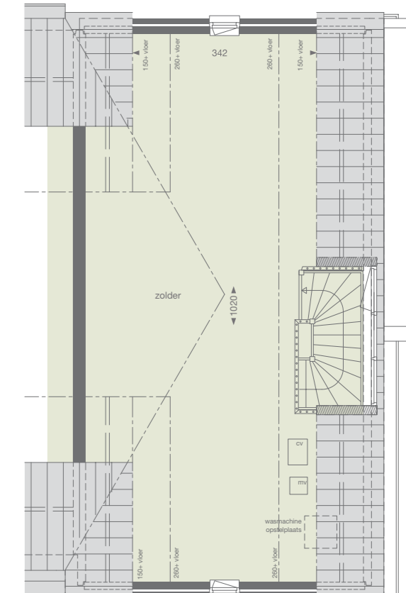
Tweede verdieping - K2
