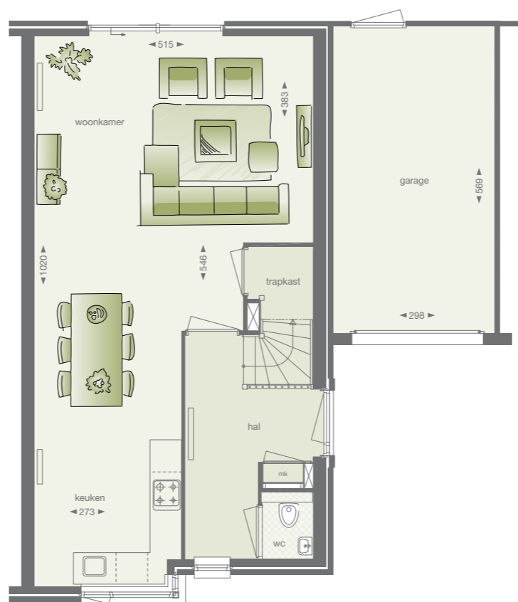
Begane grond - K1
